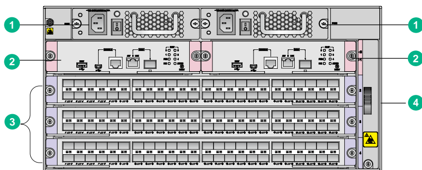
图1-1 S8600X-03-G 前面板示意图
