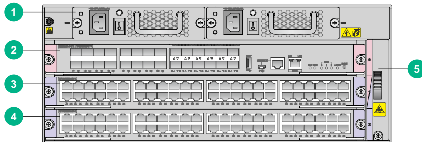
图1-2 S8600X-03M-G 前面板示意图
