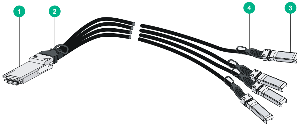
图4-9 QSFP+ to SFP+DAC 电缆示意图
