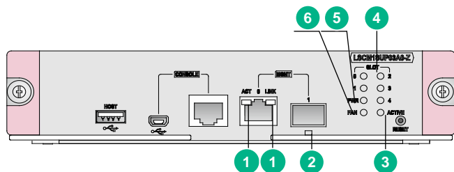
图3-1 LSCM1SUP03A0-Z 主控板指示灯示意图
