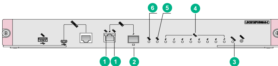
图3-2 LSCM1MPUS06A0-Z 主控板指示灯示意图
